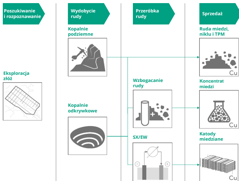
Schemat 5. Uproszczony schemat podstawowej działalności w Grupie Kapitałowej KGHM INTERNATIONAL LTD.
